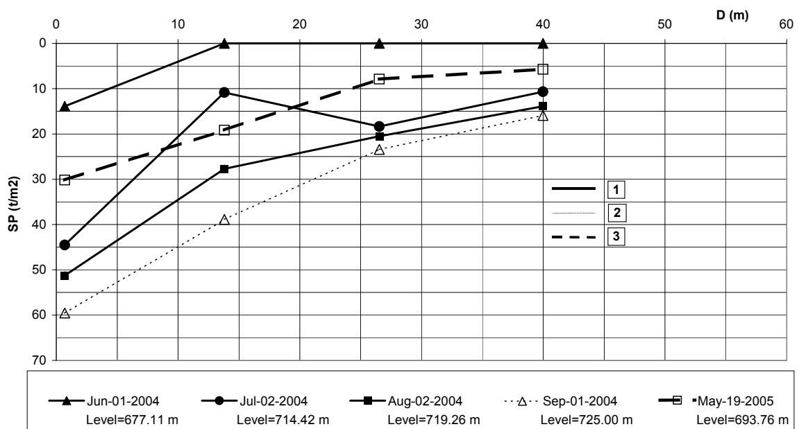
Figura 4: Historial del diagrama de subpresiones en el bloque 15. D (m) corresponde al ancho de la fundación de la presa en el bloque 15 y SP ( t/m^2 ) a la subpresión bajo el sello de fundación.
