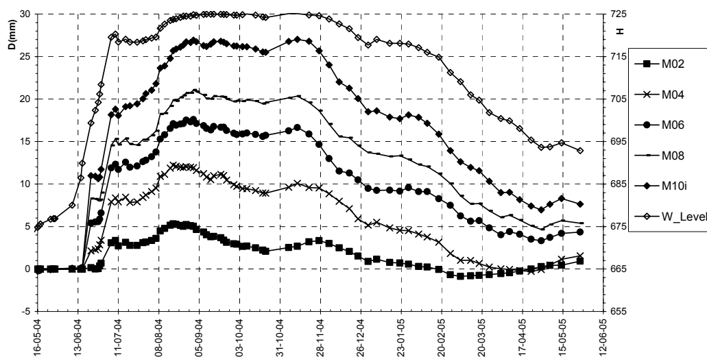
Figura 5: Desplazamientos horizontales del coronamiento.
